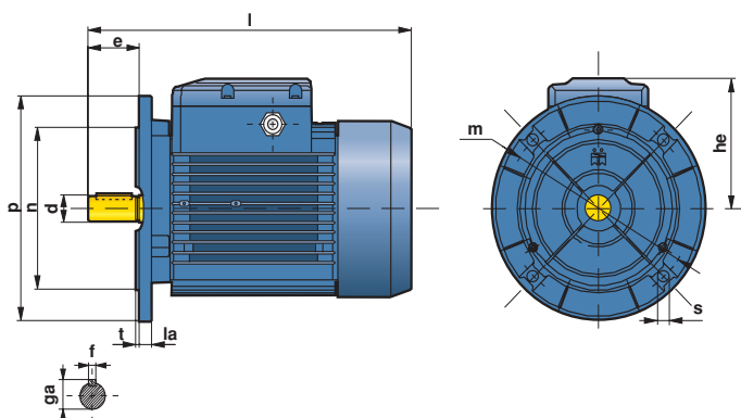
FRAME SIZE B14 (IM 3601)
