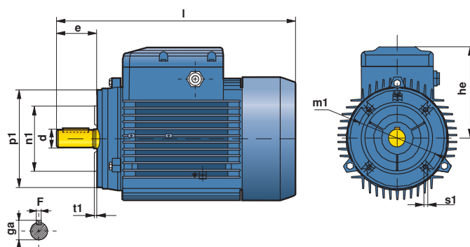
FRAME SIZE B14 (IM 3601)
